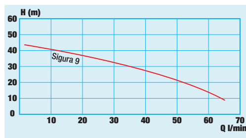
Driftskarakteristik ved 2850 min -1
